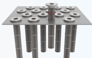
法兰和密封垫片安装
