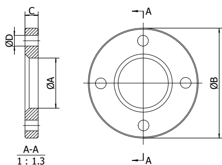
法兰结构平面图
